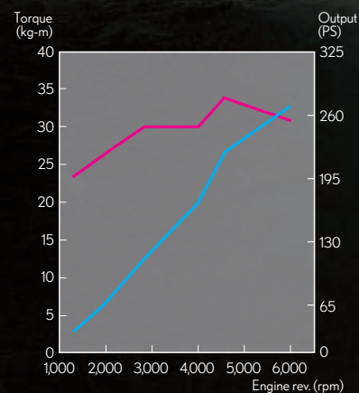
RX 450h、RX 450hL 引擎動力輸出曲線圖
