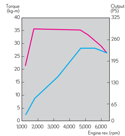
RX 300 引擎動力輸出曲線圖
